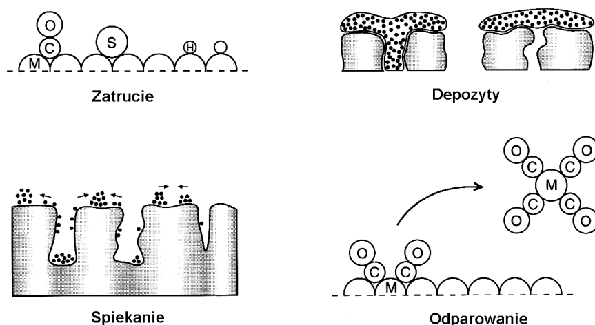
Rys. 3. Utrata aktywności katalizatora.
